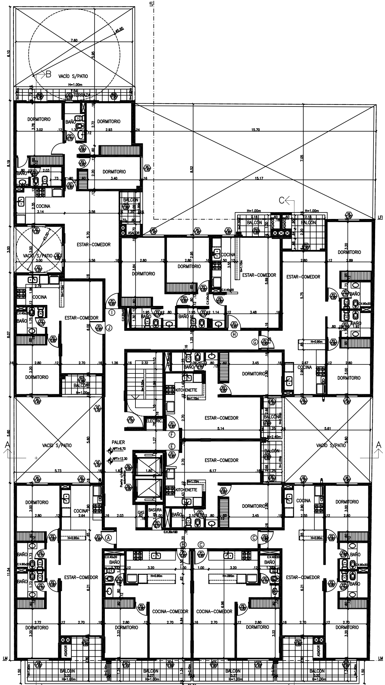
B PLANTA 5ª PISO
